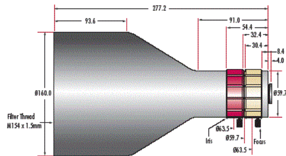
0.08X & 0.06X Telecentric Lens
