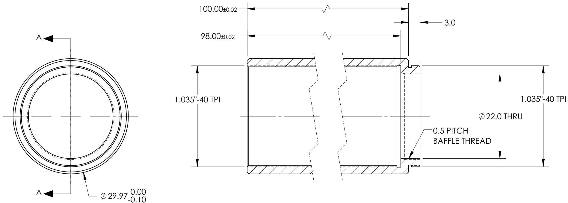
SECTION A-A
